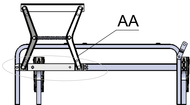
AA (1:3) Места крепления мех-ма Х5
